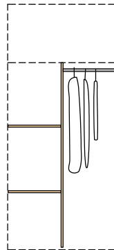
319-60 Tussenschot/2planken +1 roede HxBxD 147x52x1.6cm
